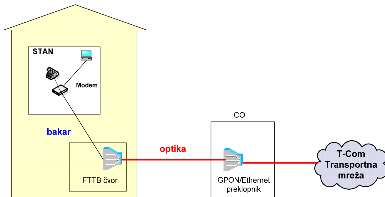
Slika 3435. Način realizacije FTTB koncepta u pristupnoj mreži
