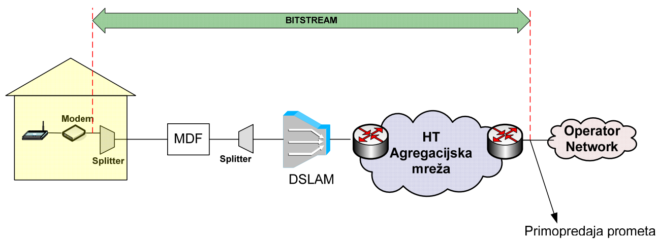
Slika 3334. Podatkovna usluga na Ethernet razini putem ADSL tehnologije
