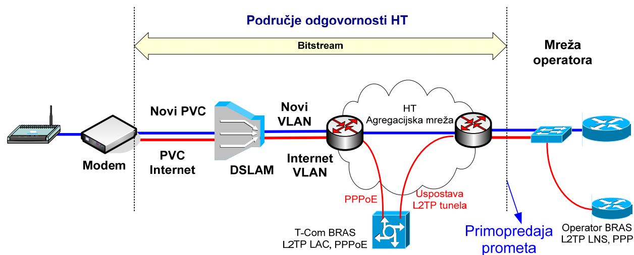
Slika 3233. Realizacija posebnog virtualnog kanala za Podatkovnu uslugu preko ADSL pristupa
